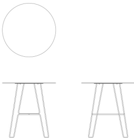
Cafe Table TUI-06 W 700 D 700 H 720
